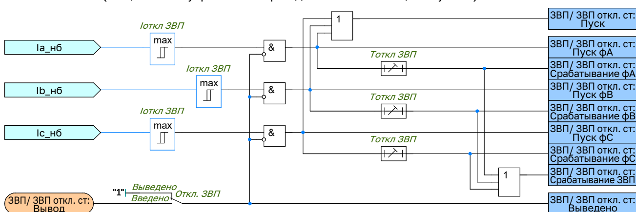
Рисунок 2.10 – Функциональная схема логики ступеней ЗВП
